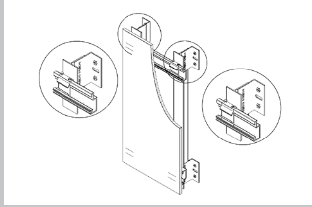
Gizli bağlantı sistemi Invisible fixing system
