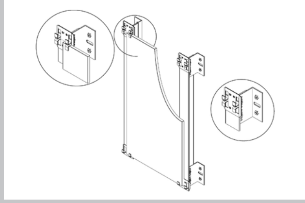
Görünür bağlantı sistemi Visible fixing system
